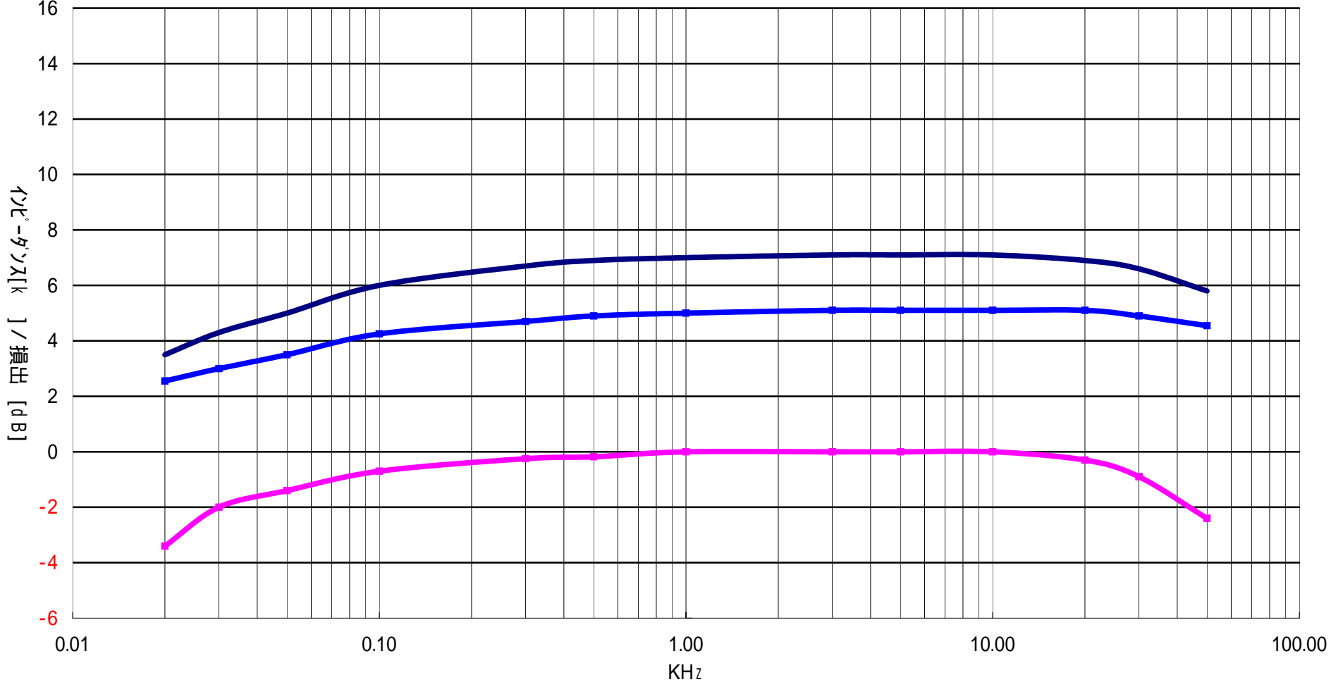
— 入力インピーダンス [K] ZP = 7K — 入力インピーダンス [K] ZP = 5K — 損出[dB]
