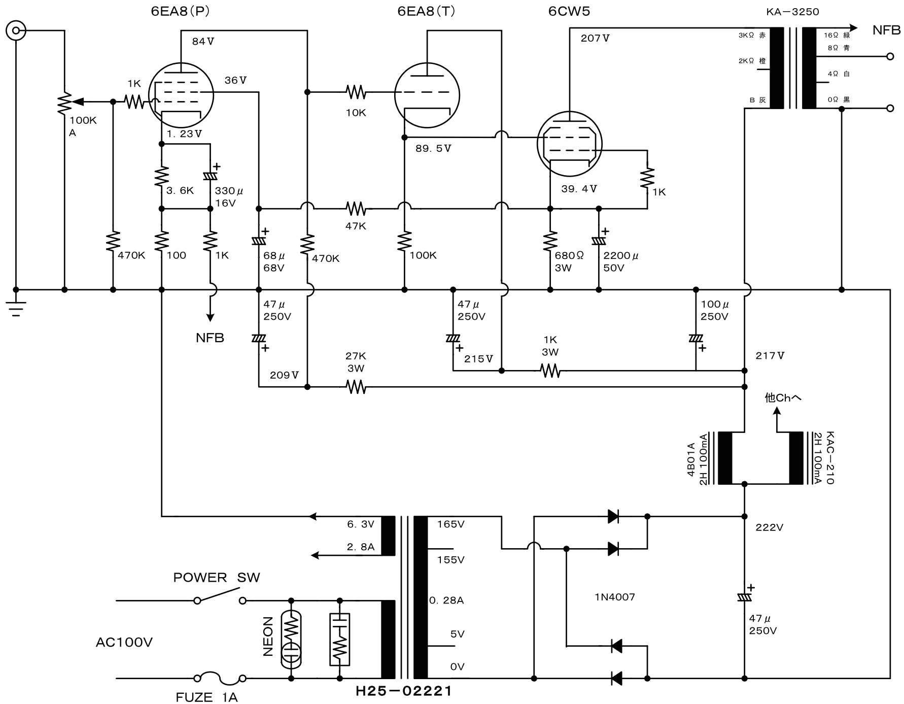
6CW5 G2ドライブ 170V動作
